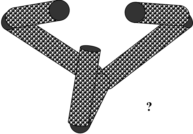
Dieses Bild soll glaube ich ein Elektron darstellen. Dies hat mir jedenfalls eine asexuelle Stimme in einem unserer Filme mal erzählt.
