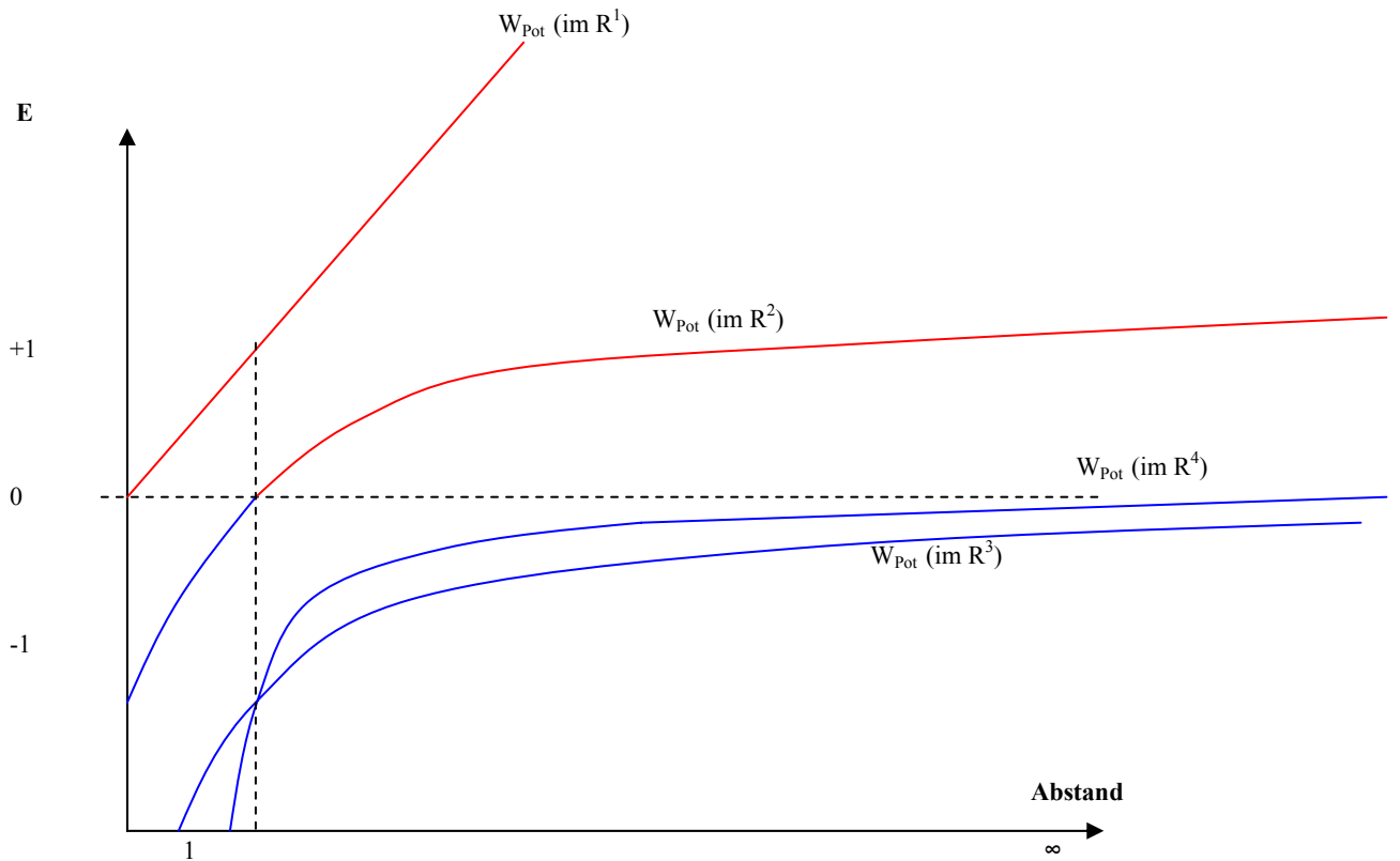
Abb.: Gravitatives Potenzial in Räumen unterschiedlicher Dimensionalität. Wie man sieht ist das Grav. -Potenzial in einem 3-dimensionalen Raum für Abstände größer 1 (genormt an der Größe eines Einheitspartikels) am Niedrigsten. Unmittelbar darüber liegen die Grav-Potenziale der Reihe nach eines 4-dim, eines 5-dim, 6-dim ..... Raumes usw. Deutlich darüber im positiven Bereich findet sich schließlich das Grav-Potenzial eines 2-dim Raumes und an oberster Stelle das Grav-Potenzial eines 1-dim Raumes.
