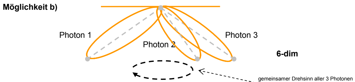
Abb.: Alle 3 Photonen befinden sich „unterhalb“ des room of interactions. Die Photonenfeldkreise 1, 2 und 3 haben einen resultierenden Drehimpuls L \neq 0 (Ein Drehsinn im Uhrzeigersinn soll resultieren).
