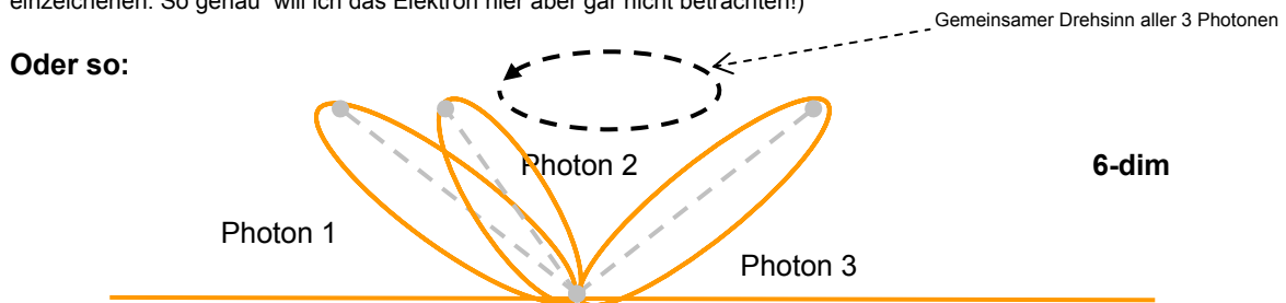
Abb.: Alle 3 Photonen befinden sich „oberhalb“ des room of interactions. Die Photonenfeldkreise 1, 2 und 3 haben einen resultierenden Drehimpuls L \neq 0 (Ein Drehsinn entgegen dem Uhrzeigersinn soll resultieren).
