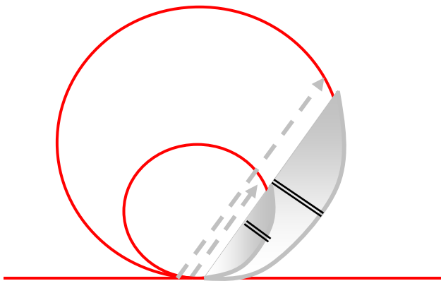
Ein "dickes" Photon, das ein kleineres schluckt?
