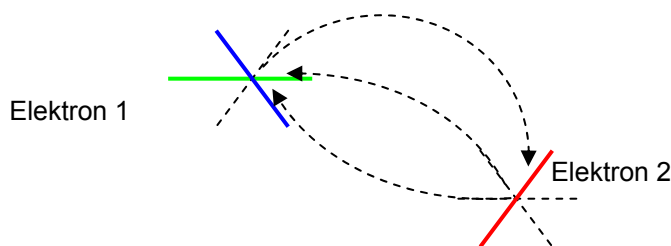
Abb.: Mögliches Meson-model: Ein dreifarbiges Photonenstrom könnte beide schweren Elektronen im Raum fixieren. Ein periodischer Wechsel von gerade von 2-farbigem oder nur einem 1-farbigem Photonenstrom im Raum fixiert, könnte periodisch nach jeweils einer Periode T wechseln. Nur in einem 3-farbigem Photonenstrom ist eine punktuelle gegenseitige Fixierung im Raum möglich. Agglomerationen aus solcherart gebundenen spin \frac{1}{2} Teilchen sollten daher besonders stabil sein.
