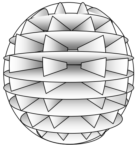
der zwei-ebnige Äther
