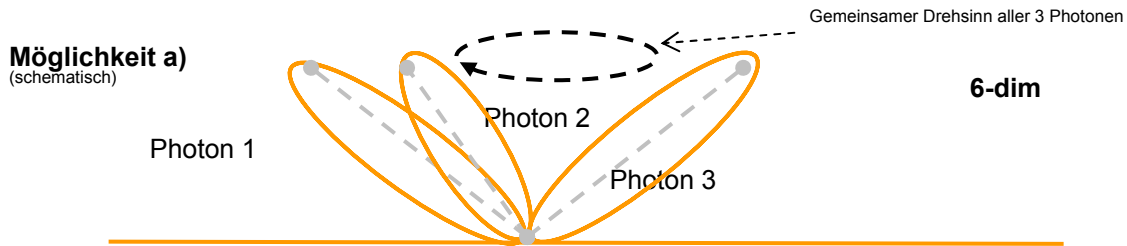
Abb.: Alle drei Photonen befinden sich „oberhalb“ des flachen room of interactions (durchgezogene orange Linie). Die Photonenfeldkreise 1, 2 und 3 haben einen resultierenden Drehimpuls L \neq 0 (Drehsinn im Uhrzeigersinn). (Genaugenommen muss man eigentlich auch noch die 3 großen gepunkteten äußeren virtuellen Photonenfeldkreise einzeichnen. So genau will ich das Elektron hier aber gar nicht betrachten!)
